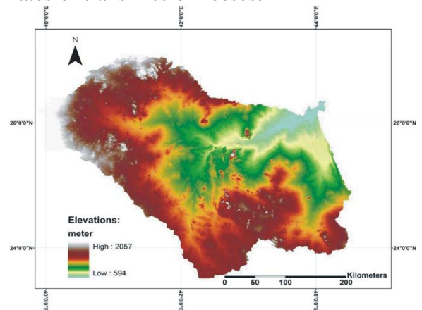
Fig. 4 : DEM of Wadi Al Rimah catchment
